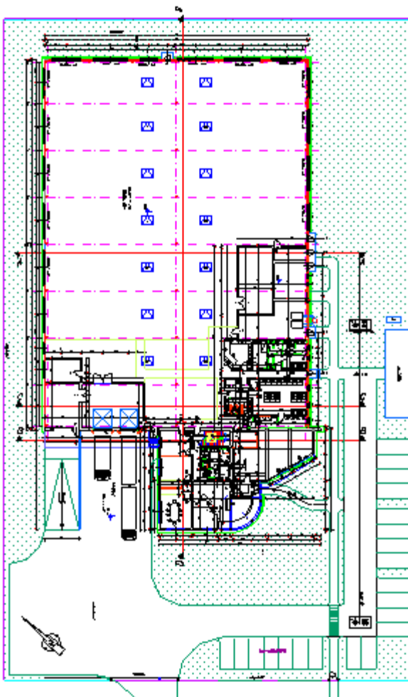
Grundrissplan EG mit Außenanlagen
