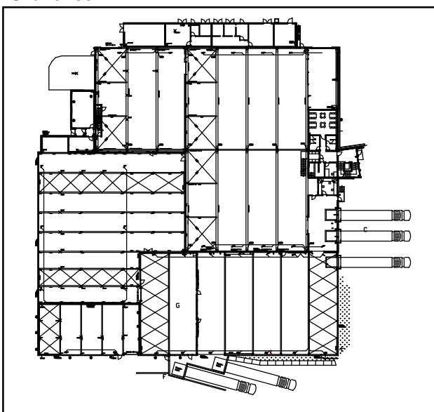
Grundriss
